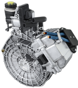
48-Volt-Netz Schaeffler
