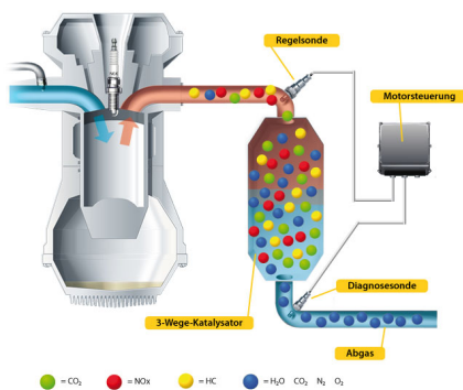
Lambdaregelkreis
