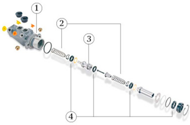
Tandem-Hauptbremszylinder: 1 Gehäuse | 2 Federn | Kolben | 4 Manschetten | Quelle: Robert Bosch GmbH
