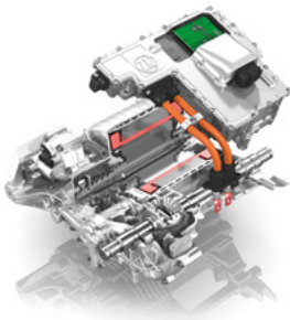
Leistungselektronik beim Elektromotor
